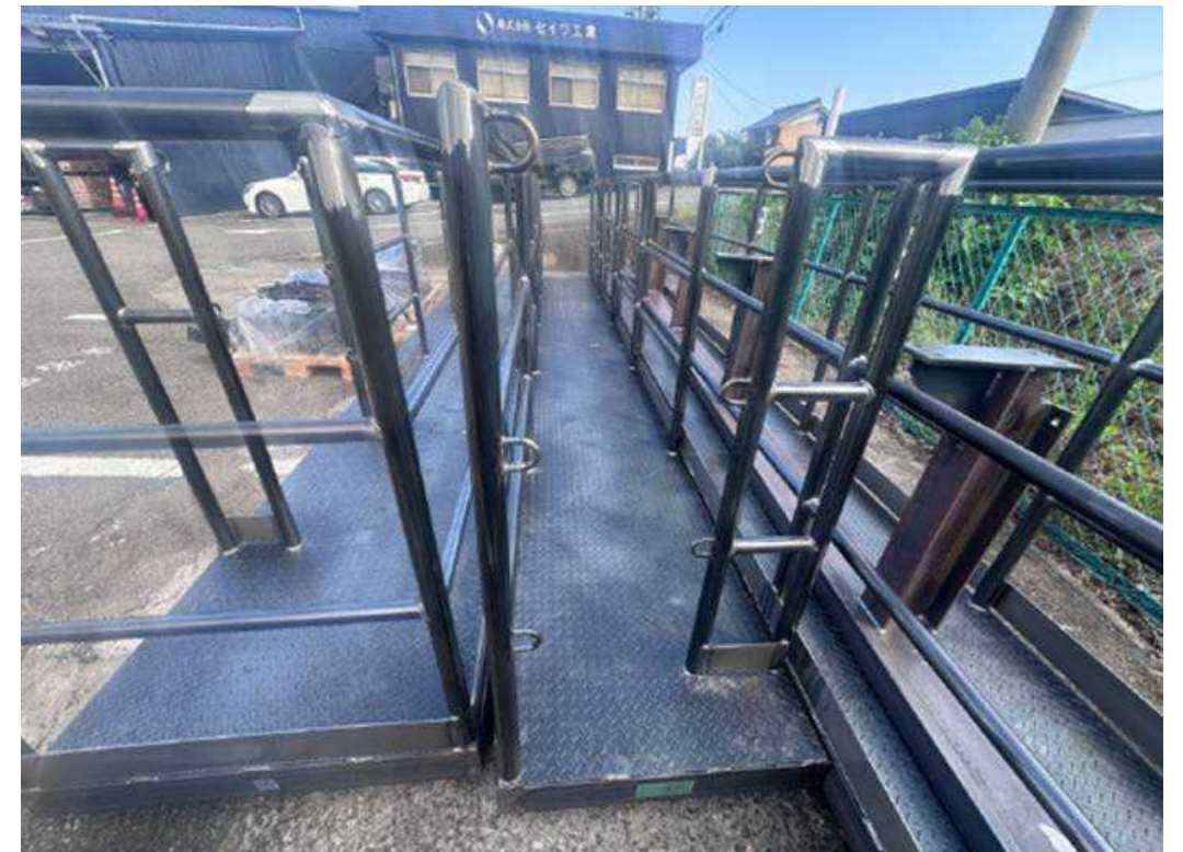
プラント歩廊手摺一体型
